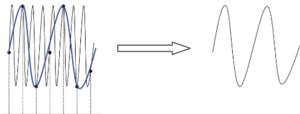
图 29 波形混叠
