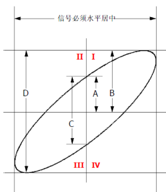
图 22 李沙育测量原理图
