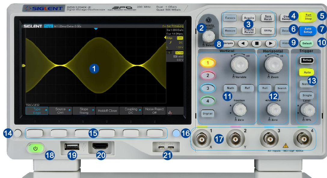
图 9 SDS1000X-E (4 通道) 机型前面板总览
