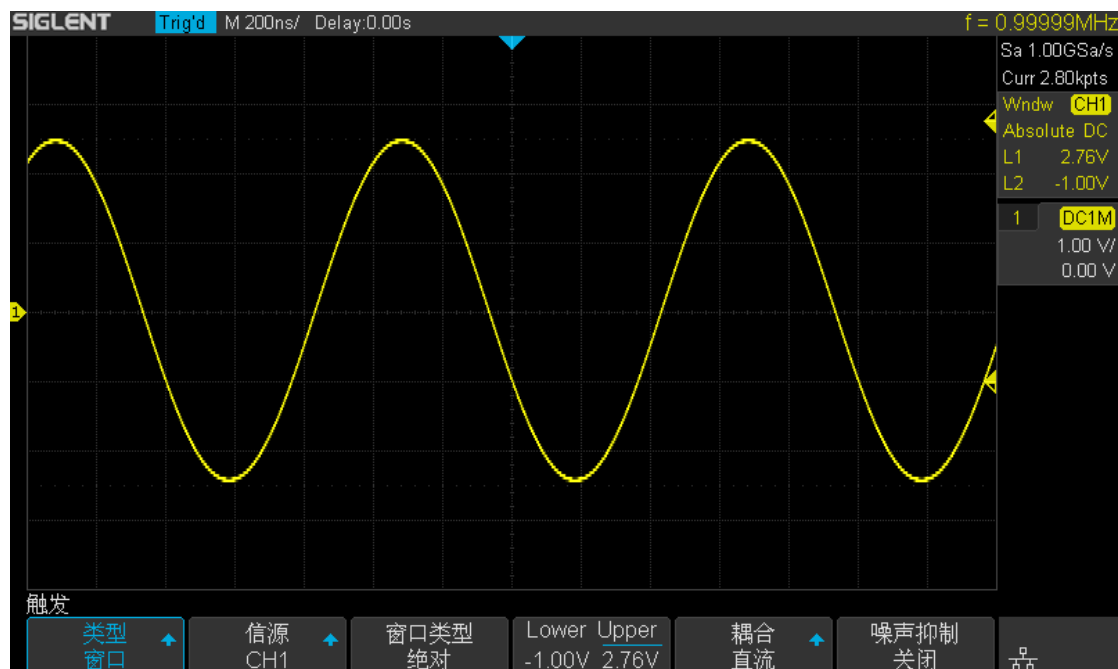
图 44 “绝对”窗口触发
