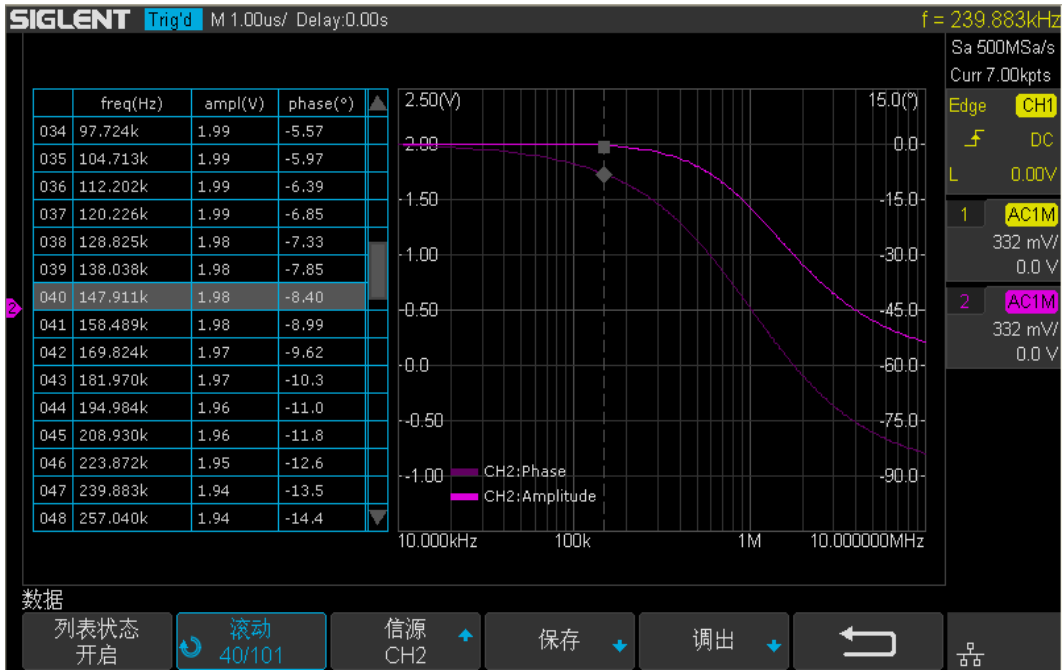
图 166 波特图列表
