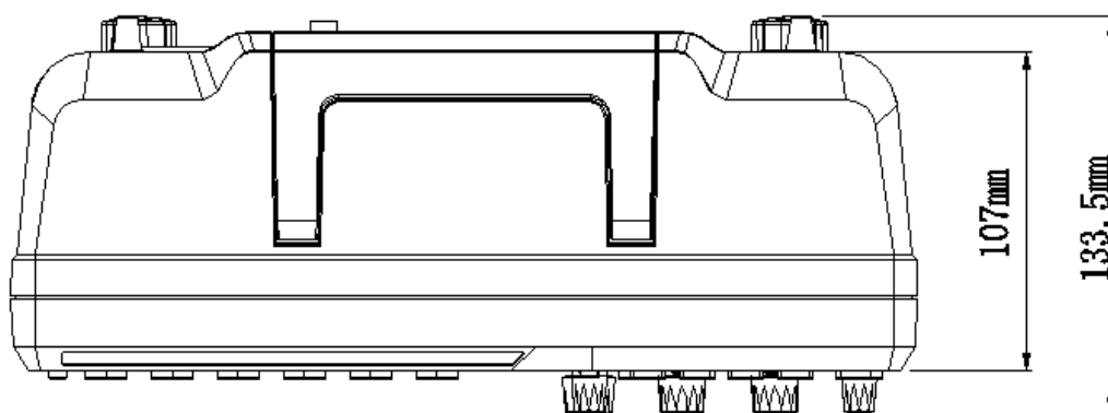
图 2 2 通道机型侧视图
