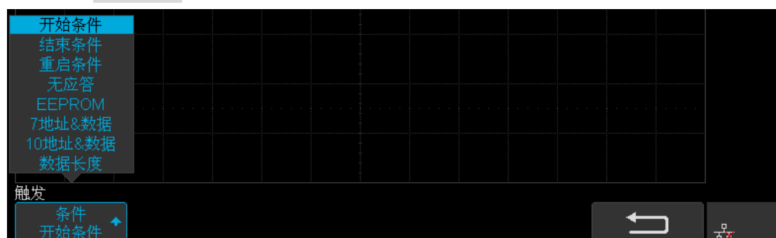
图 54 I2C 触发条件
