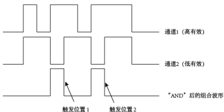
图 50 码型触发示意图
