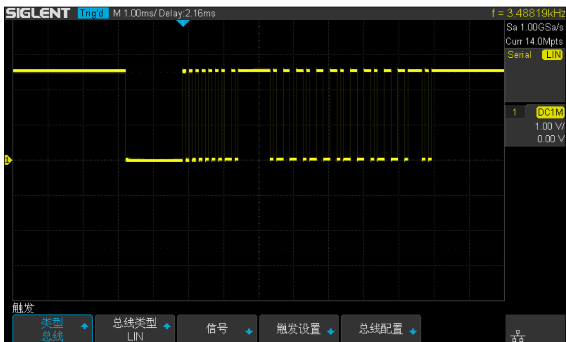
图 83 LIN 触发
