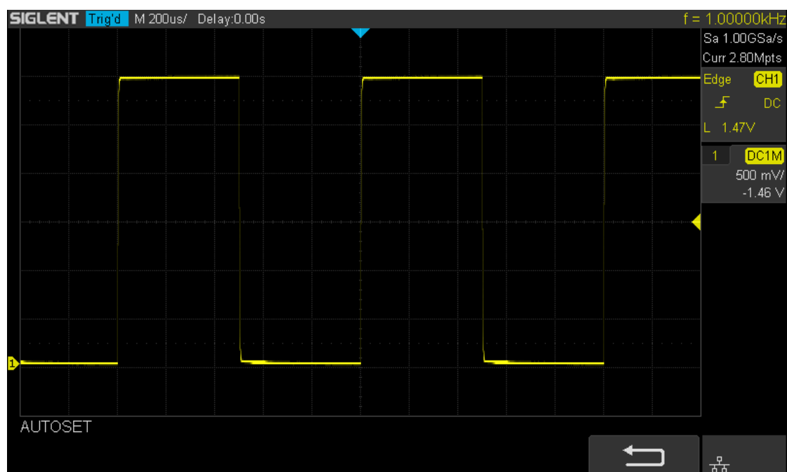
图 7 功能检查
