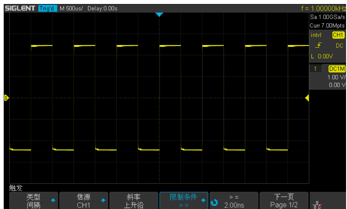
图 46 间隔触发
