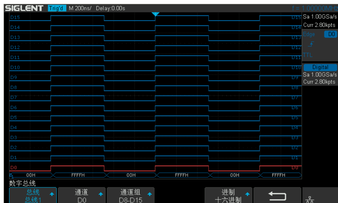
图 129 数字总线
