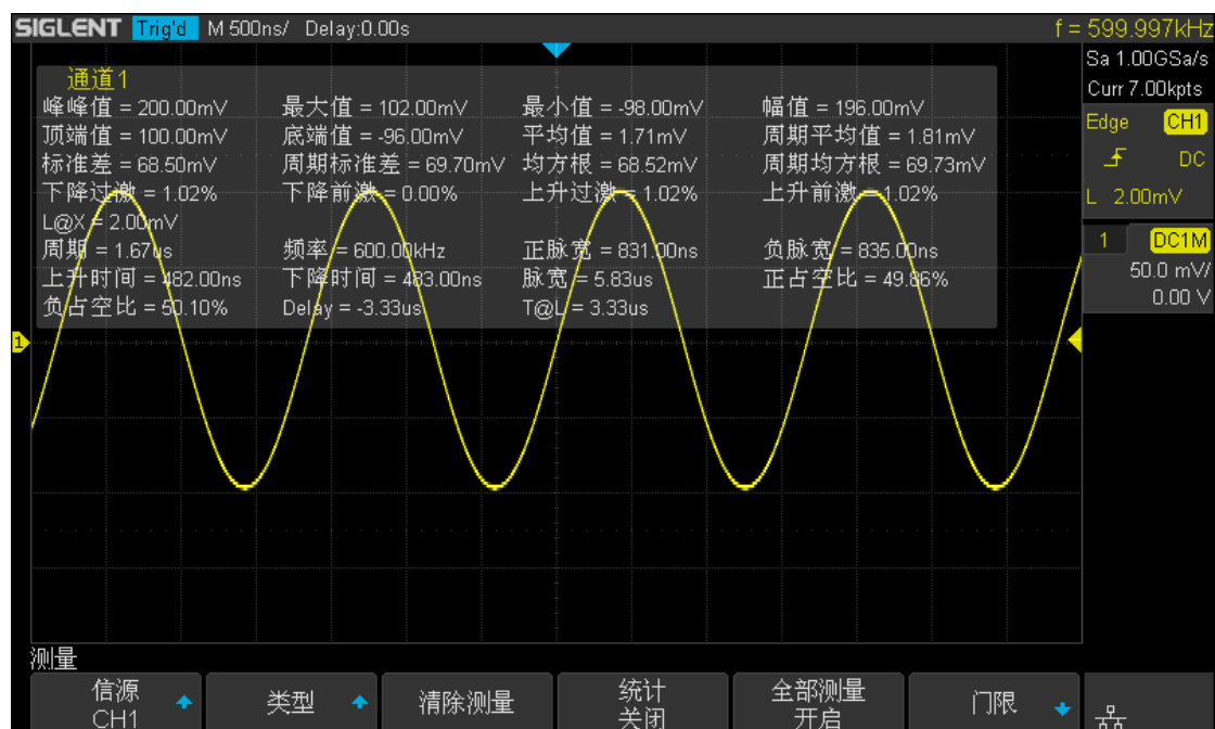
图 112 全部测量
