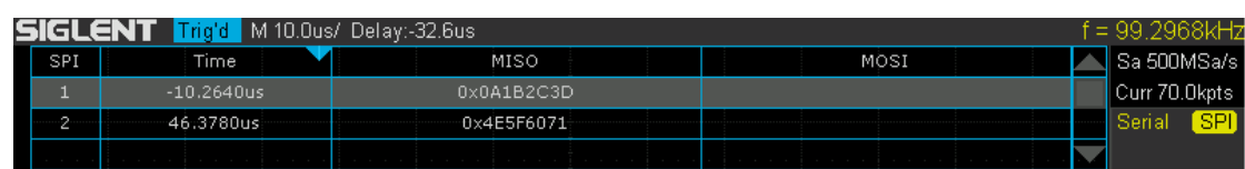
图 66 SPI 解码列表显示
