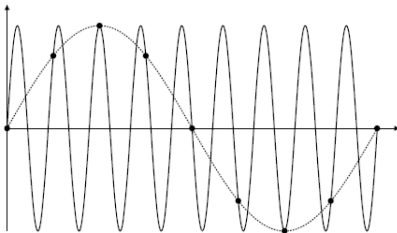
图 25 采样混叠
