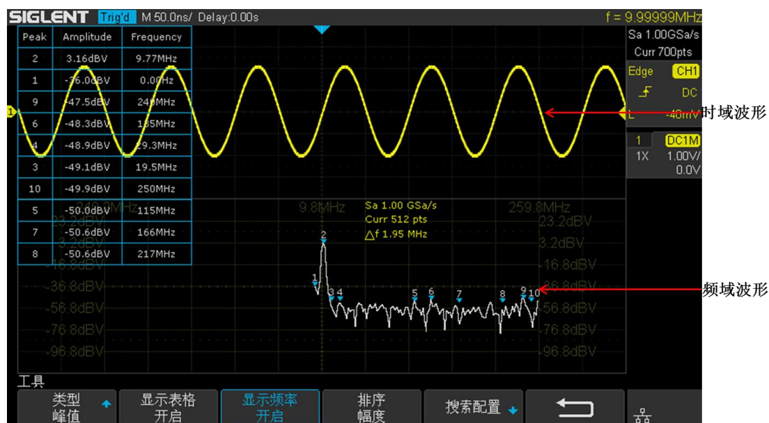
图 98 FFT 波形
