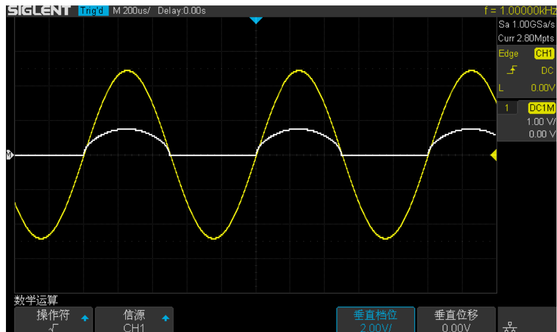
图 102 平方根运算
