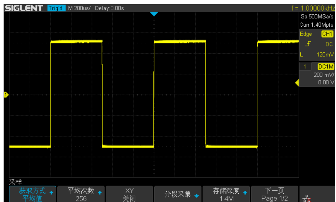
图 35 平均次数为 256 时的波形（降低随机噪声）
