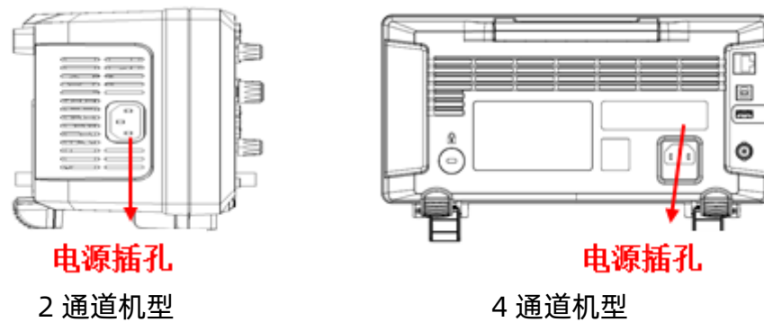
图 6 连接电源
