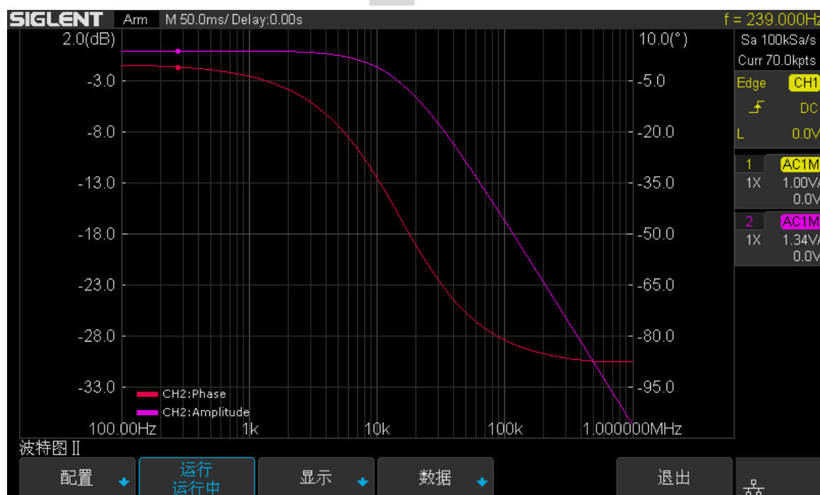
图 172 恒定幅值下波特图扫描曲线
