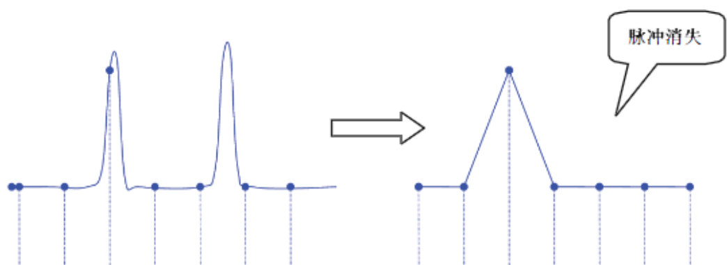
图 30 波形漏失
