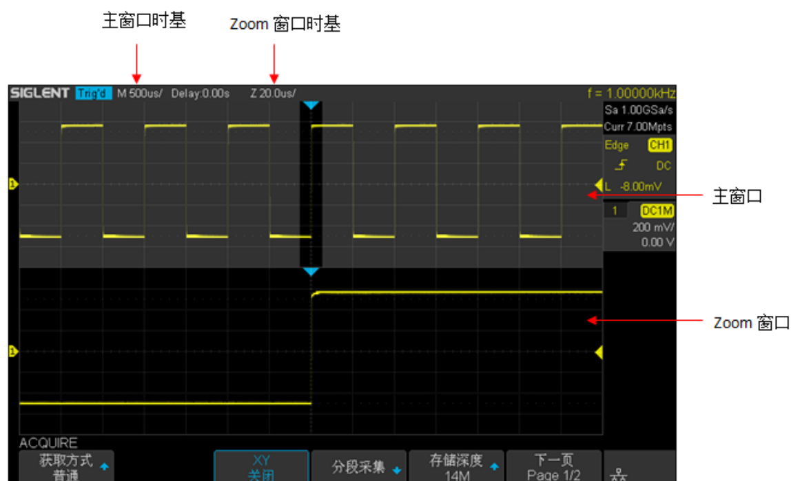
图 24 分屏缩放
