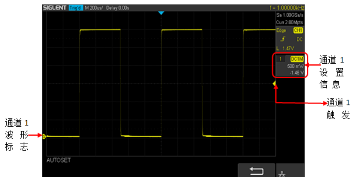
图 17 垂直通道图
