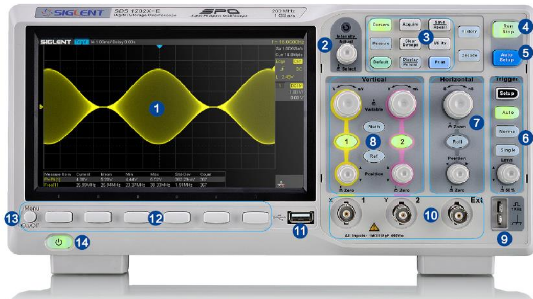
图 8 SDS1000X-E (2 通道) 机型前面板总览
