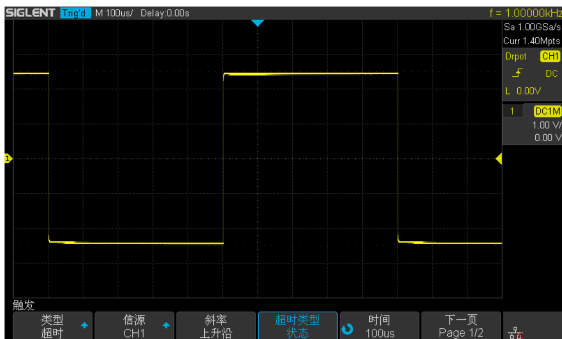
图 48 “状态”超时触发
