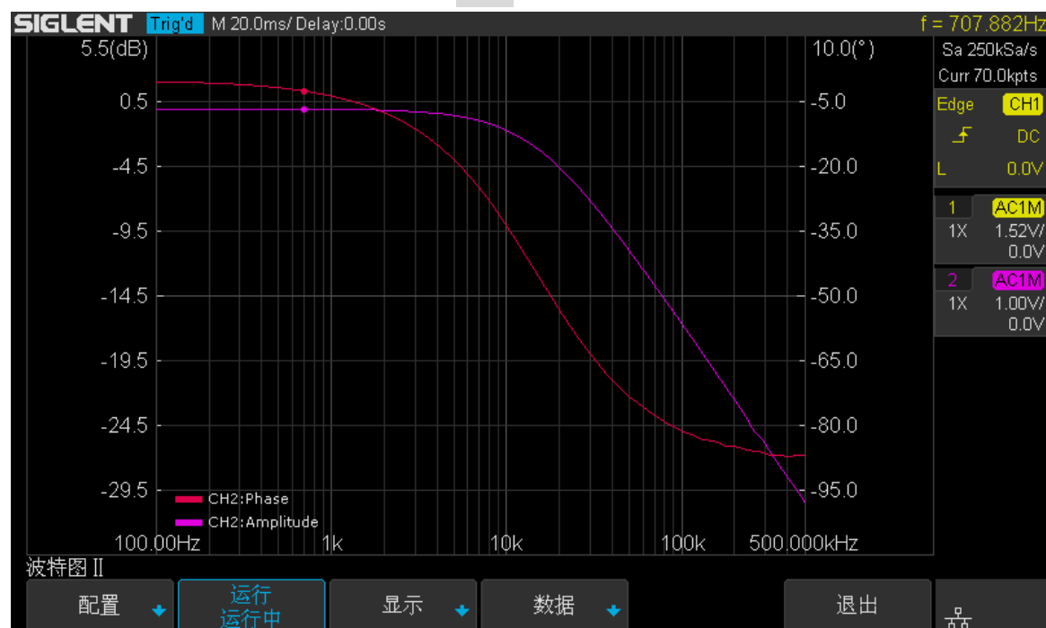
图 177 可变幅值下波特图扫描曲线
