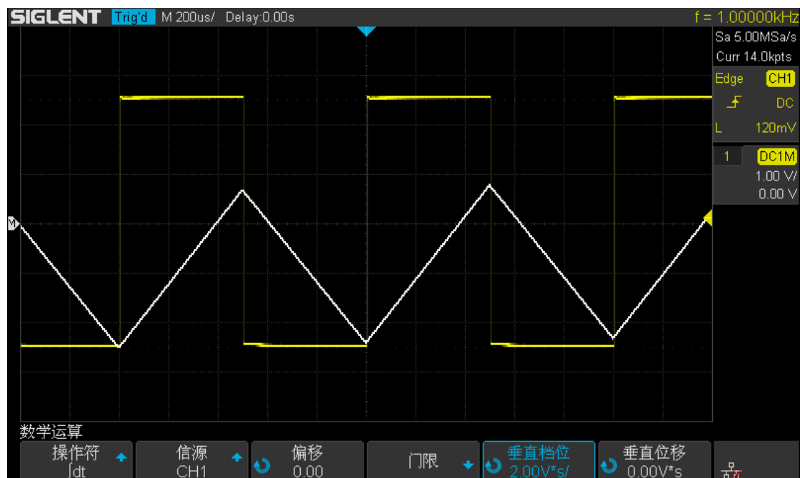
图 100 无 DC 偏移校正（积分运算）
