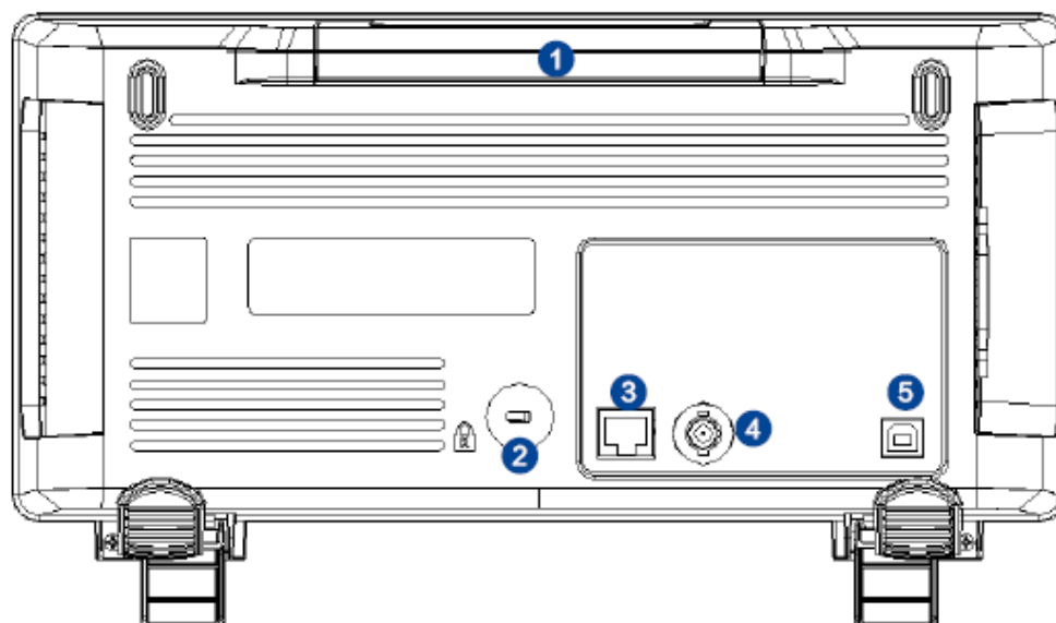
图 11 SDS1000X-E (2 通道) 机型后面板总览
