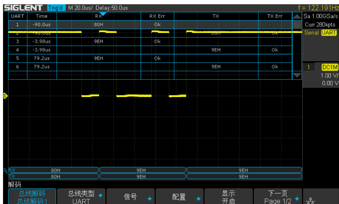
图 73 UART 解码图
