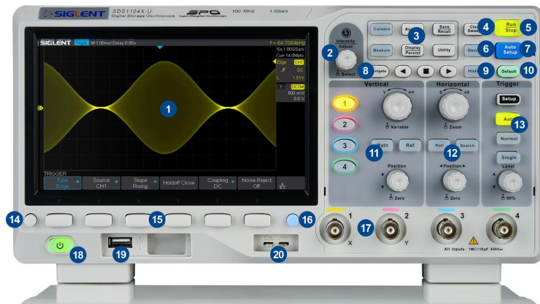
图 10 SDS1000X-U 机型前面板总览
