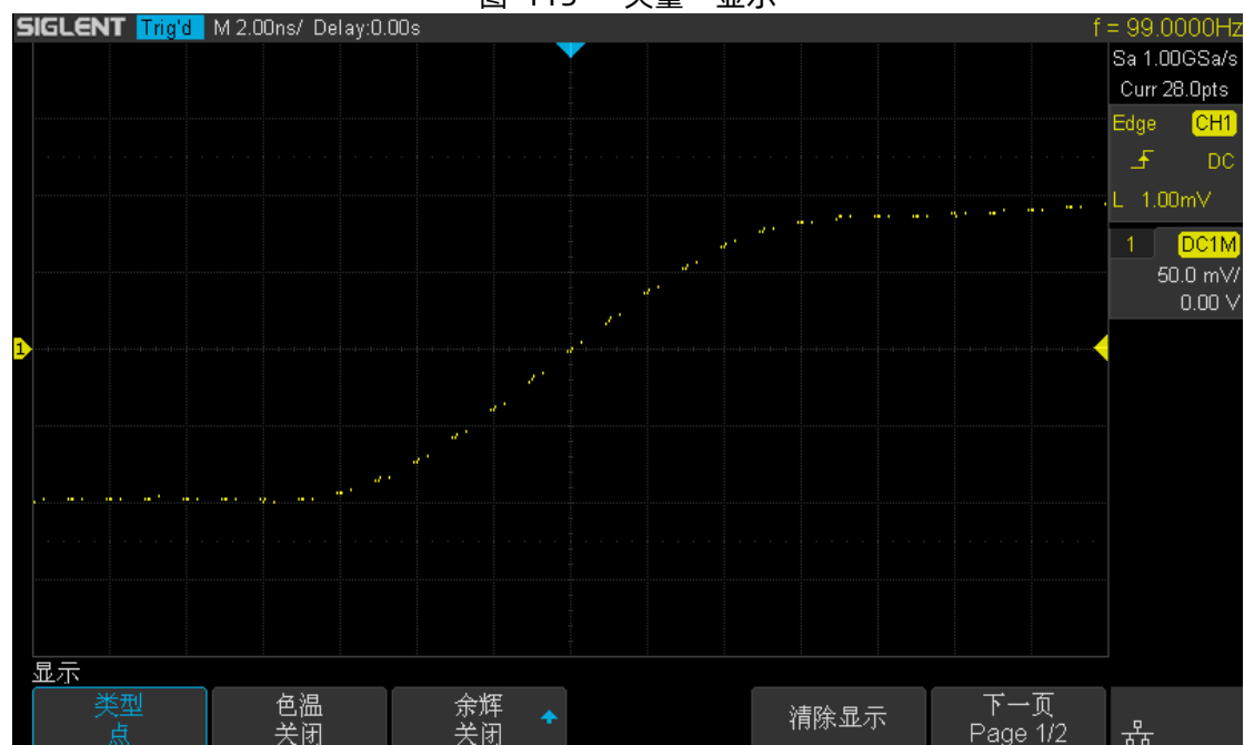
图 116 “点”显示
