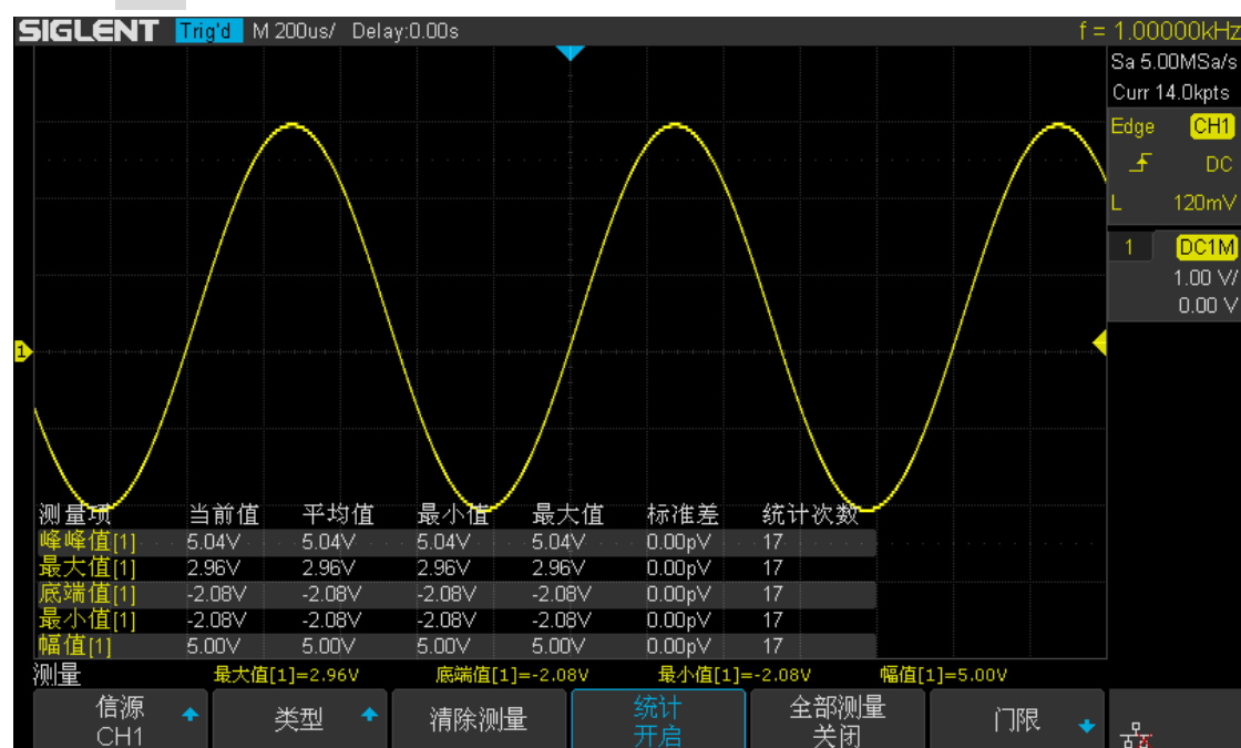
图 111 测量统计
