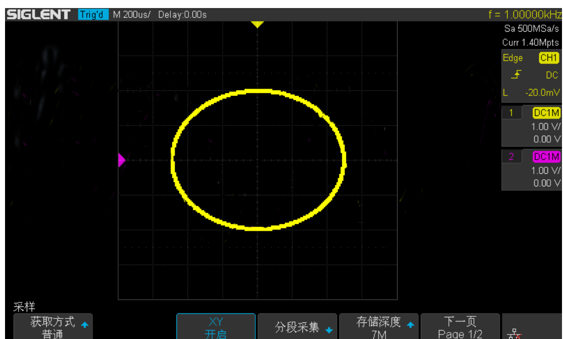
图 23 李沙育测量实例
