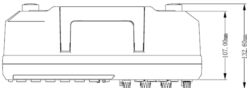
图 4 4 通道机型正视图
