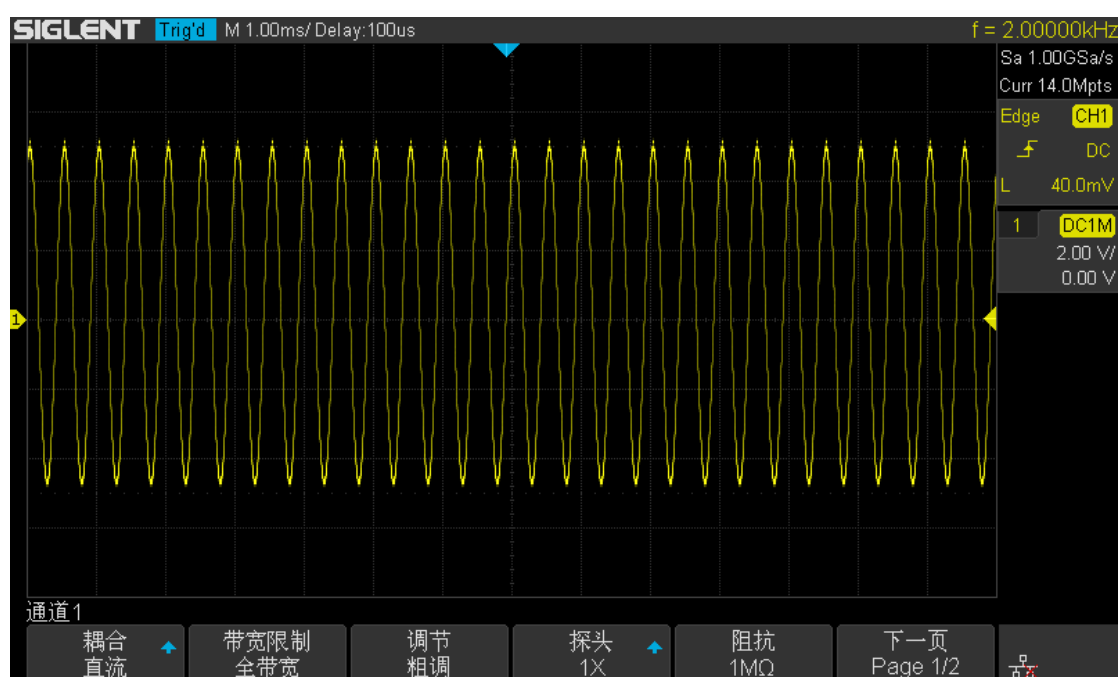
图 20 带毛刺的正弦波
