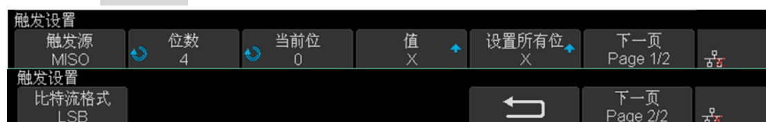
图 63 SPI 触发设置菜单
