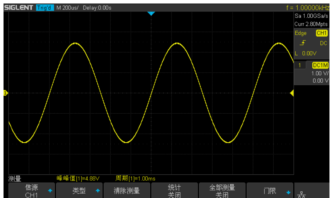
图 104 一键测量
