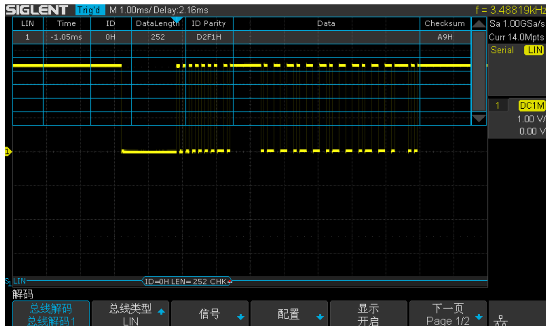
图 84 LIN 解码
