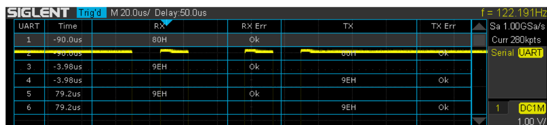
图 75 UART 解码列表显示
