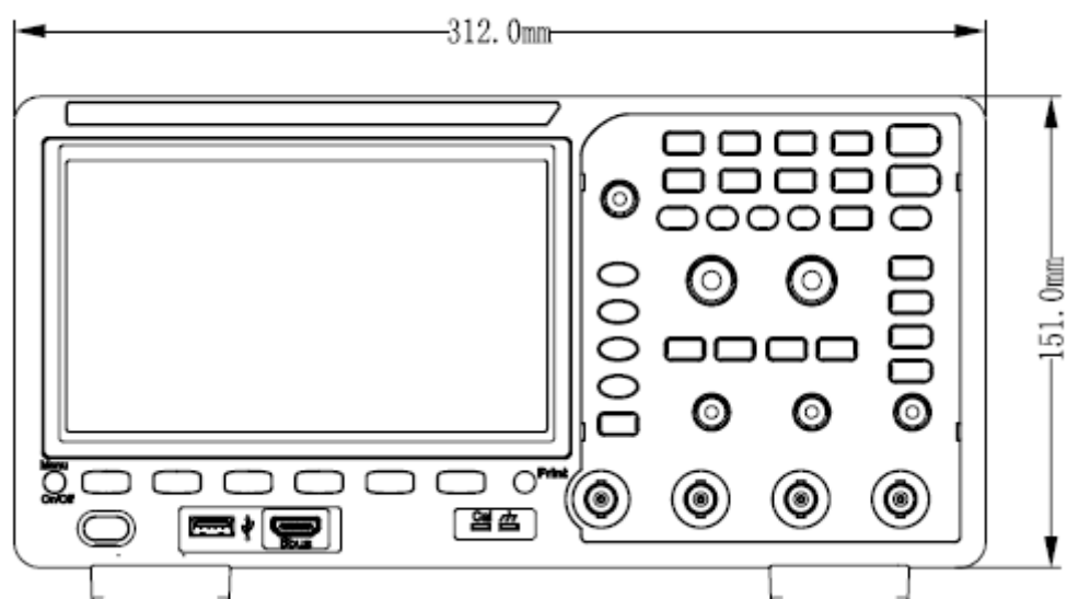
图 3 4 通道机型正视图
