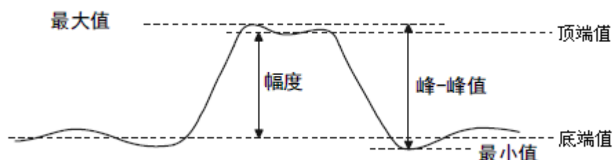
图 106 电压参数示意图
