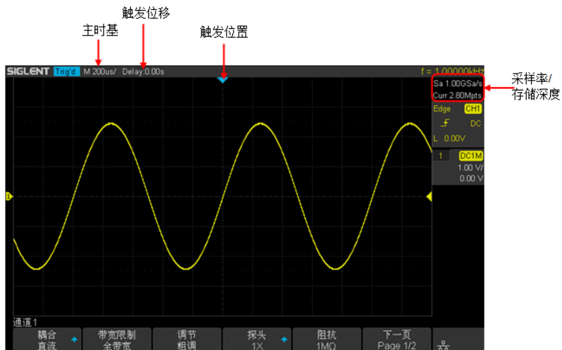
图 19 水平控制
