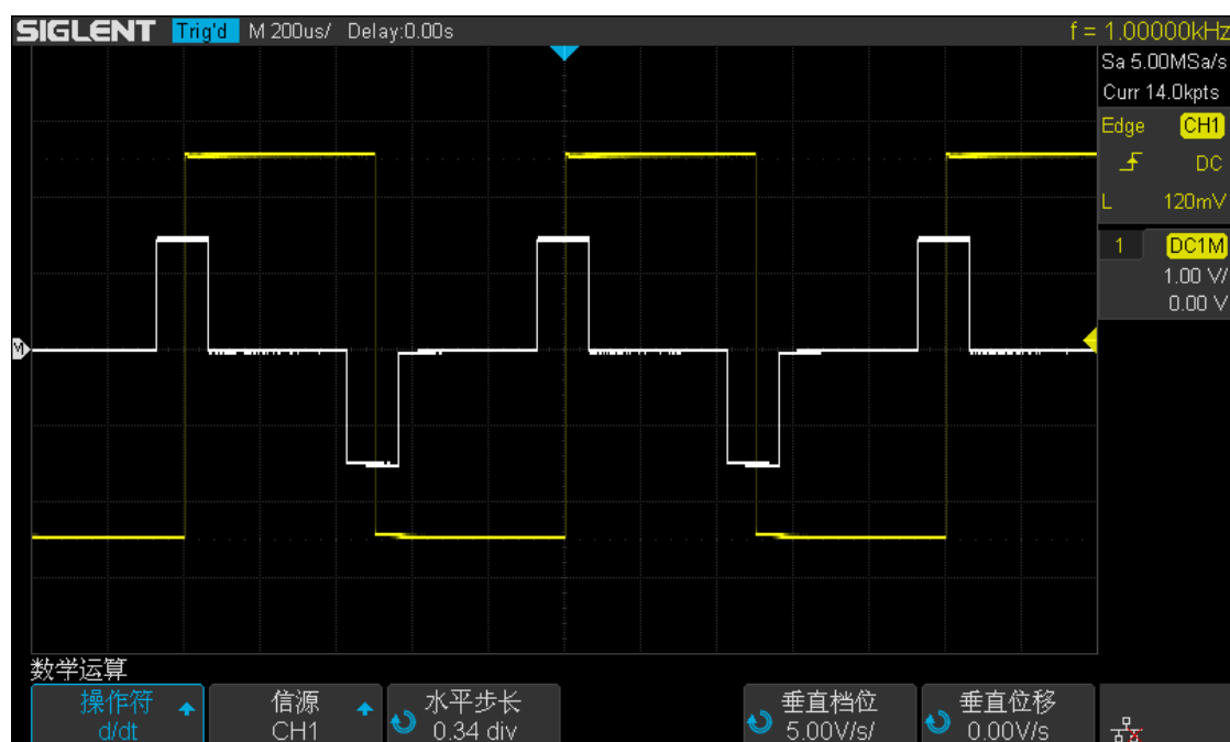
图 99 微分运算
