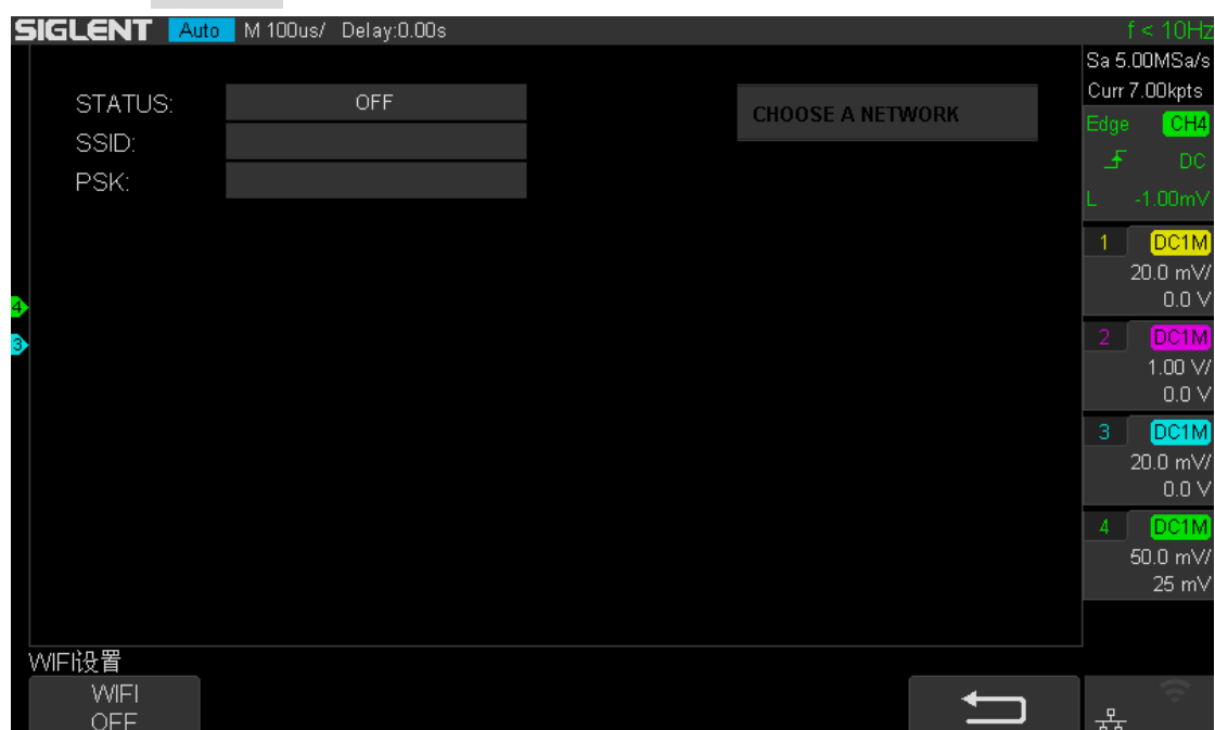
图 138 WIFI 设置界面
