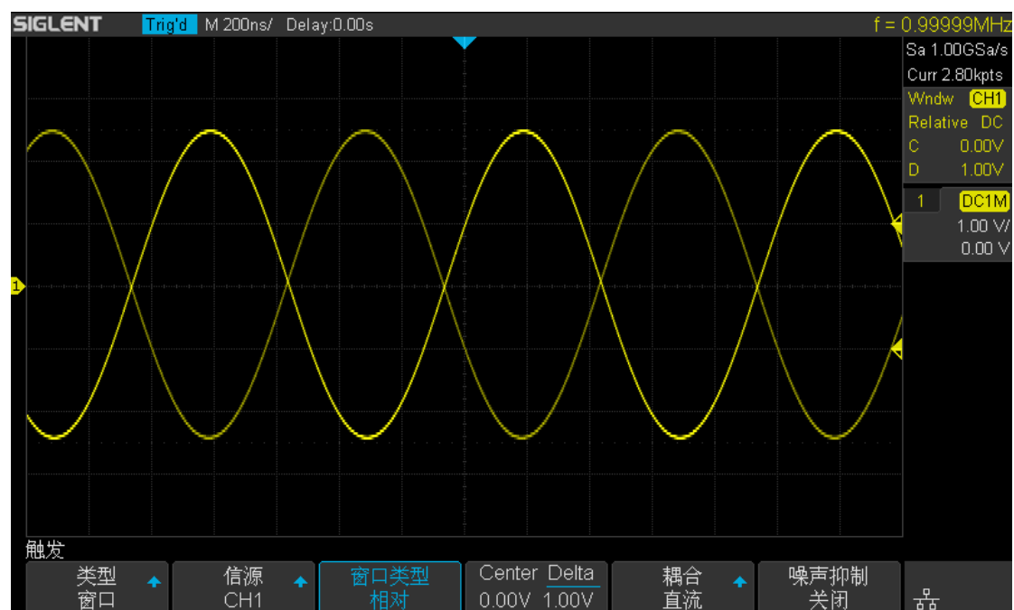
图 43 “相对”窗口触发
