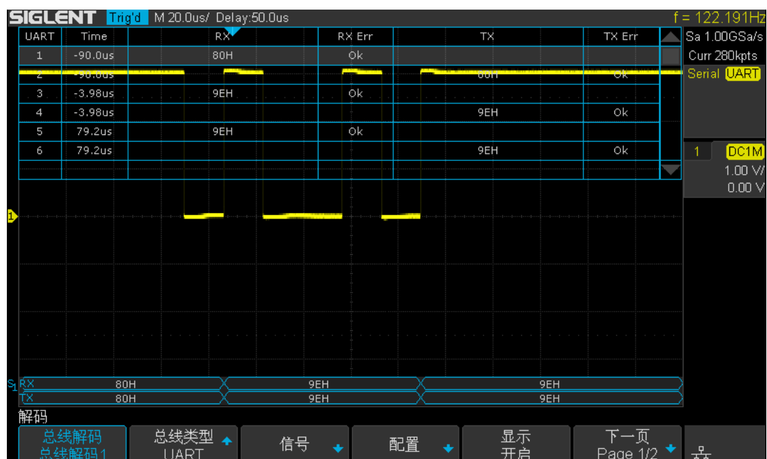
图 71 UART 解码图
