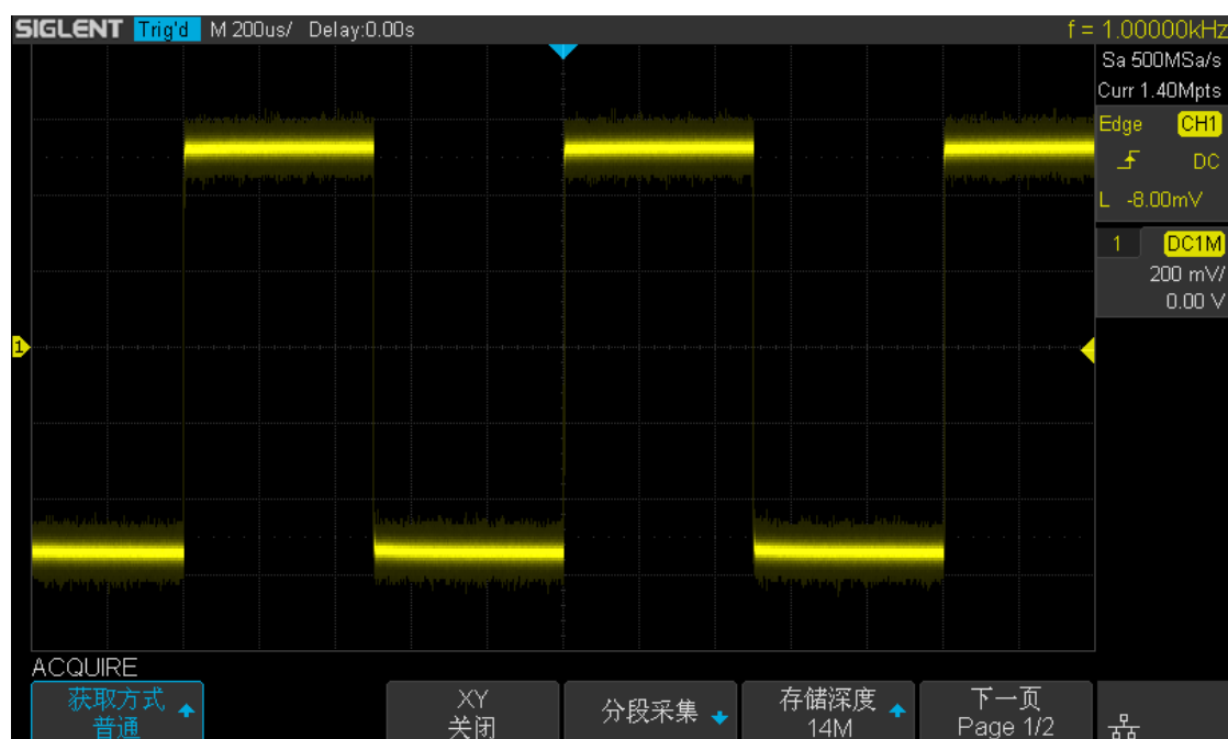
图 32 未平均时的波形（显示波形上的随机噪声）
