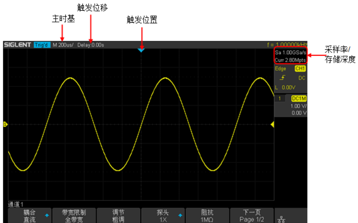
图 17 水平控制
