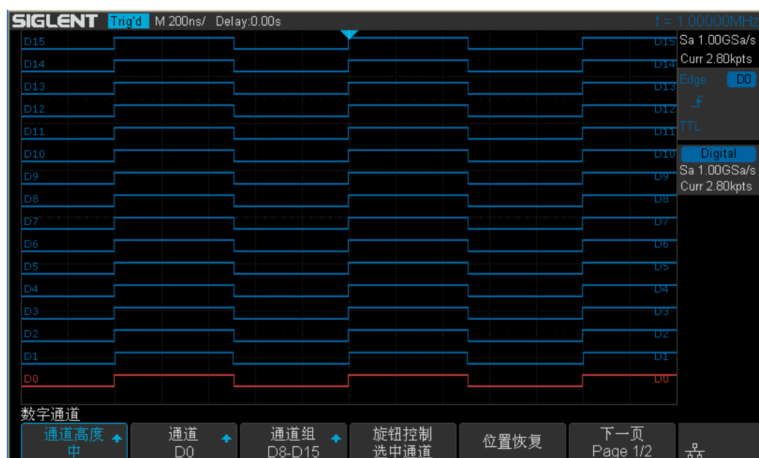
图 122 通道高度选择中
