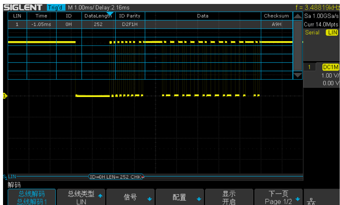
图 82 LIN 解码
