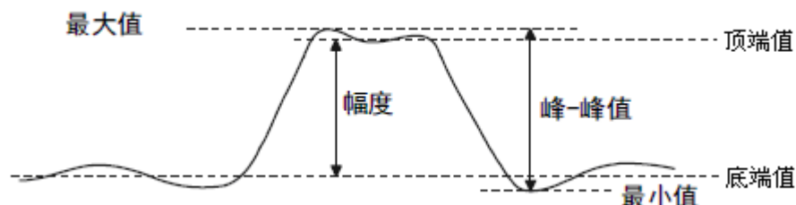
图 104 电压参数示意图
