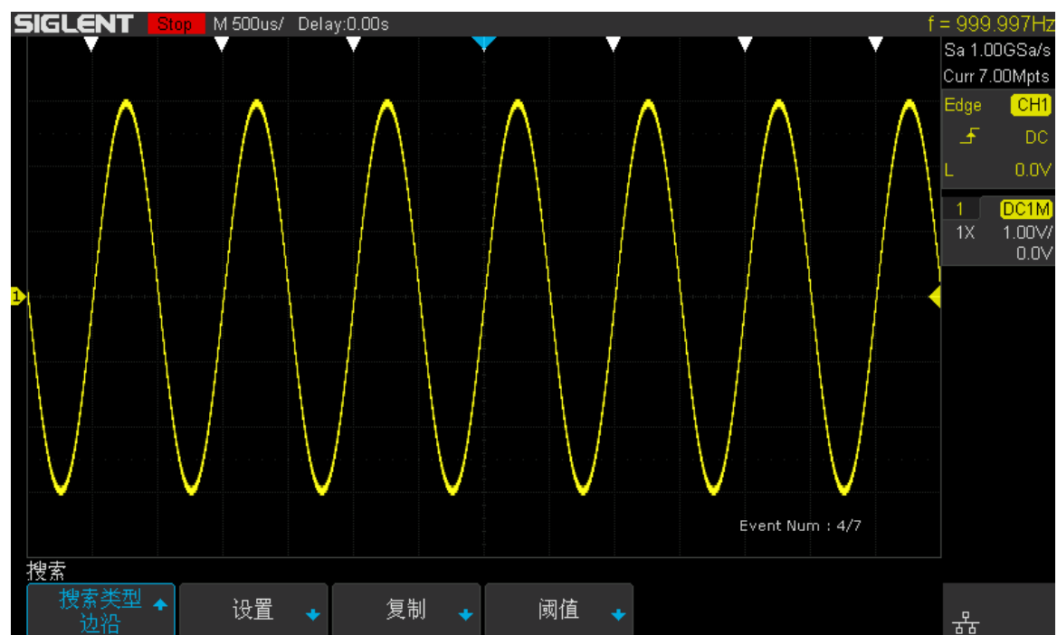
图 154 停止状态下搜索结果显示
