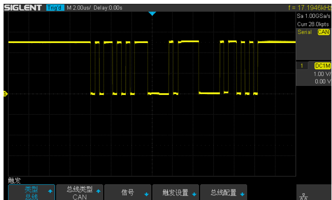
图 76 CAN 触发
