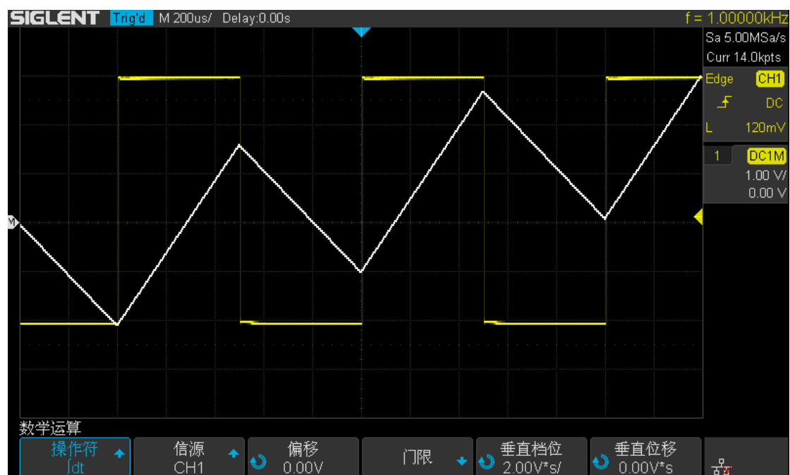
图 99 有 DC 偏移校正（积分运算）
