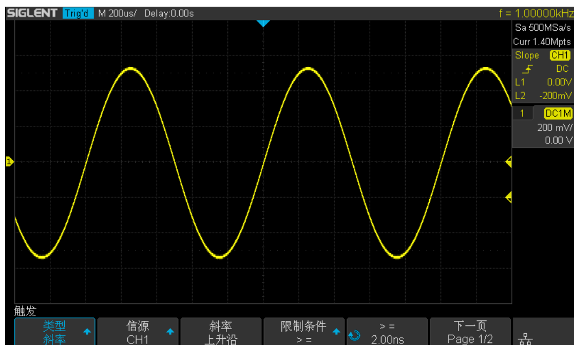
图 39 斜率触发
