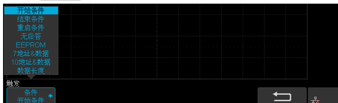
图 52 I2C 触发条件
