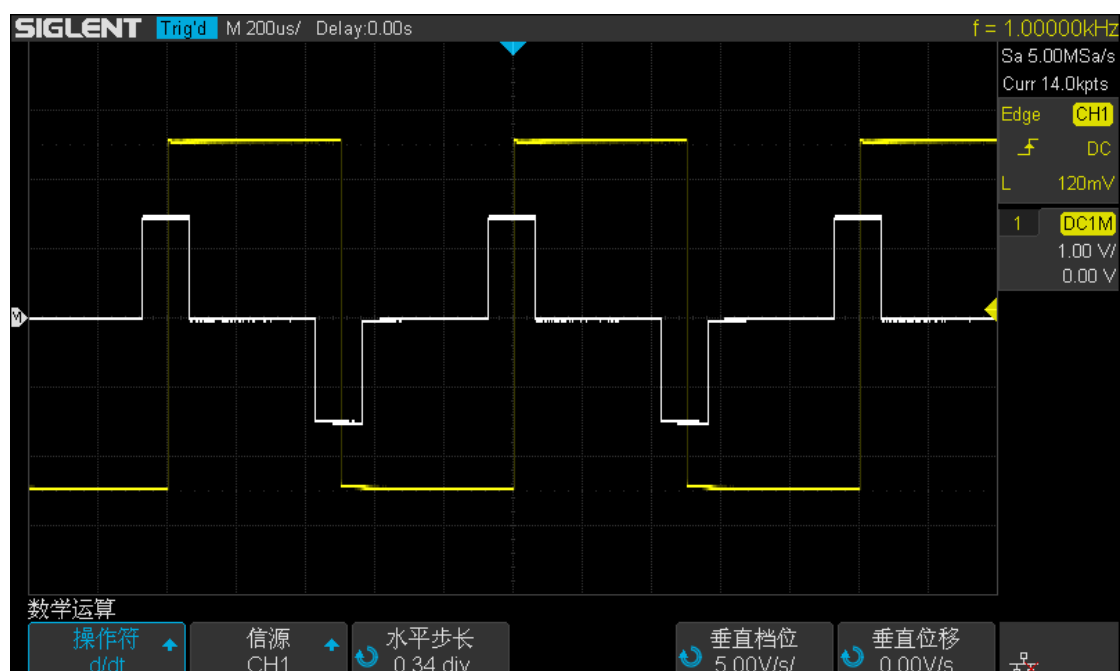
图 97 微分运算
