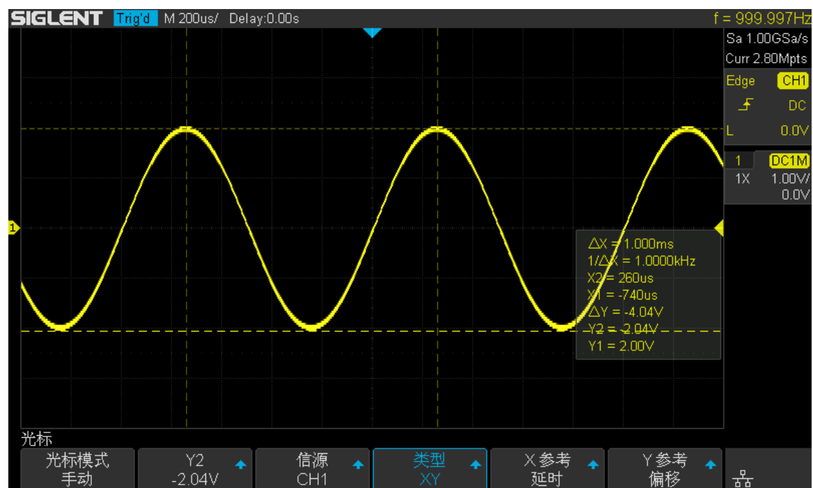
图 101 光标测量
