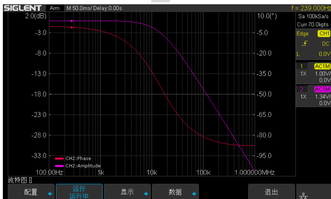
图 169 恒定幅值下波特图扫描曲线
