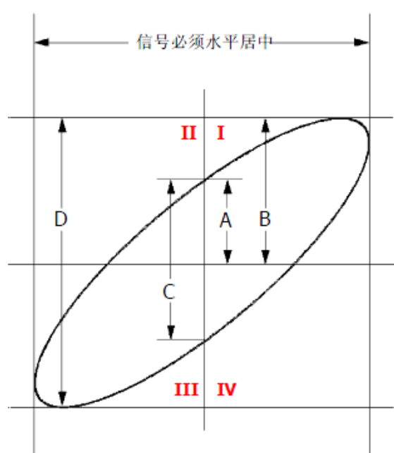
图 20 李沙育测量原理图
