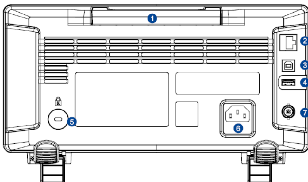
图 11-4 通道机型后面板总览
