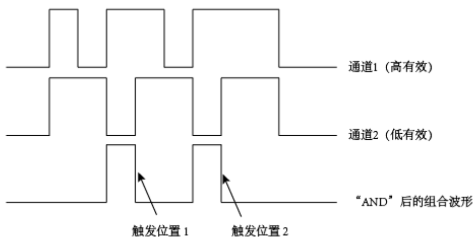
图 48 码型触发示意图
