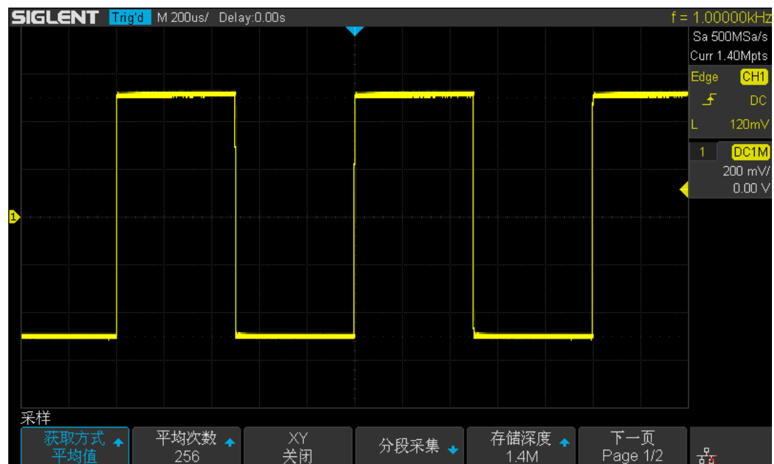
图 33 平均次数为 256 时的波形（降低随机噪声）
