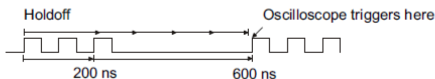
图 35 设置触发释抑时间
