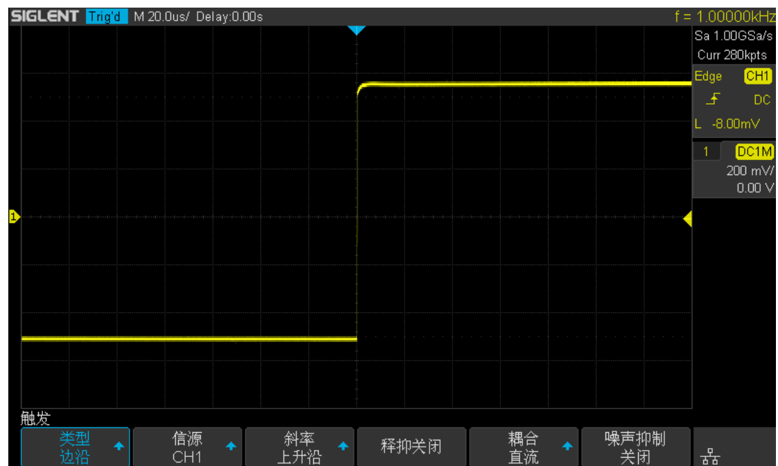
图 38 边沿触发
