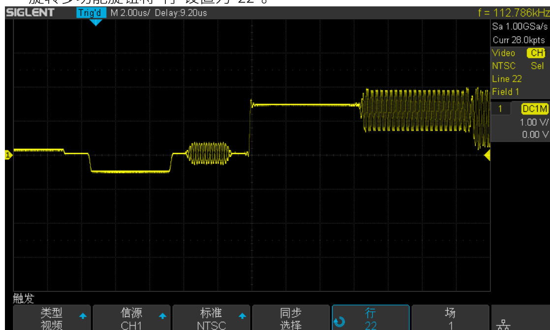
图 41 特定行上视频触发
