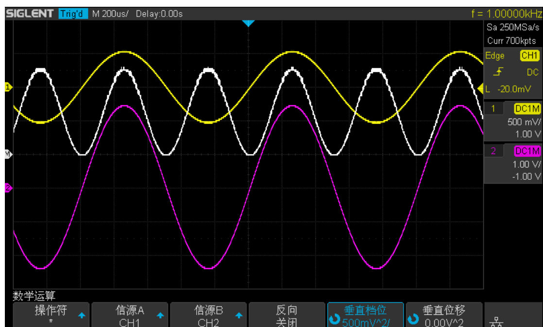
图 87 通道 1 波形乘以通道 2 波形
