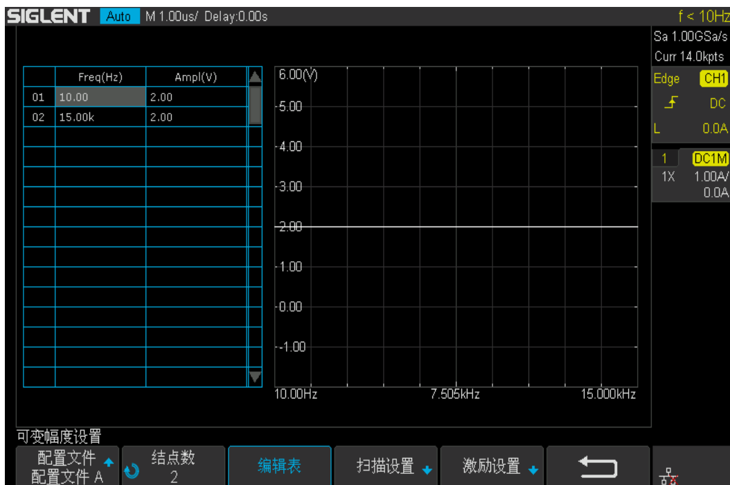
图 160 可变幅度设置
