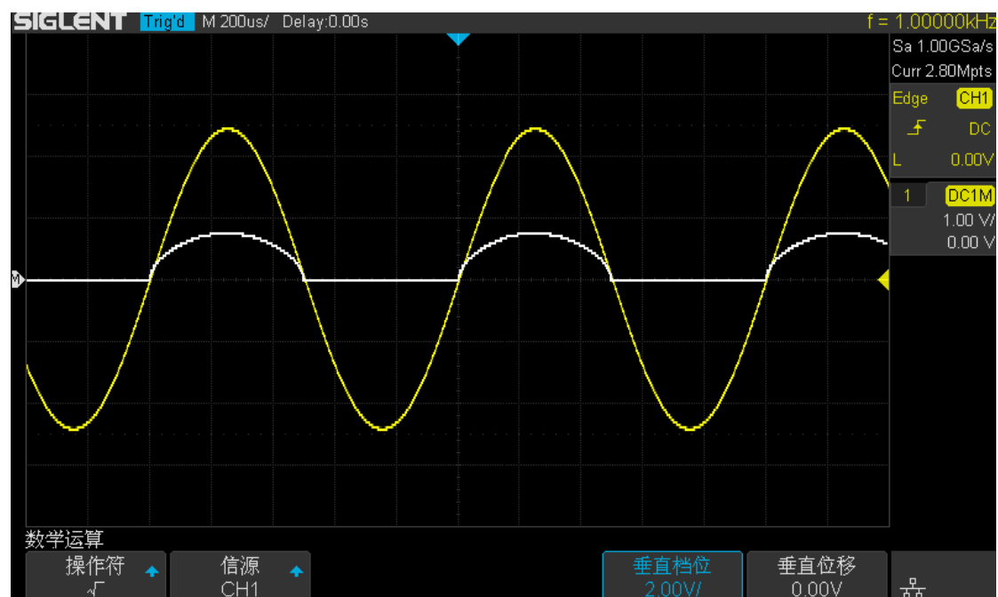
图 100 平方根运算
