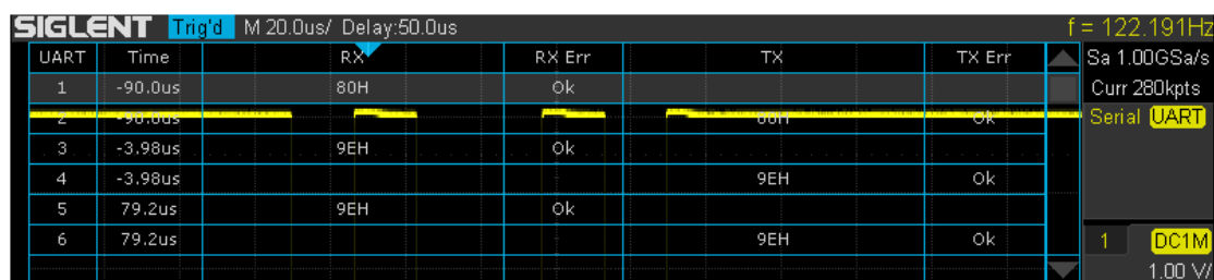
图 73 UART 解码列表显示
