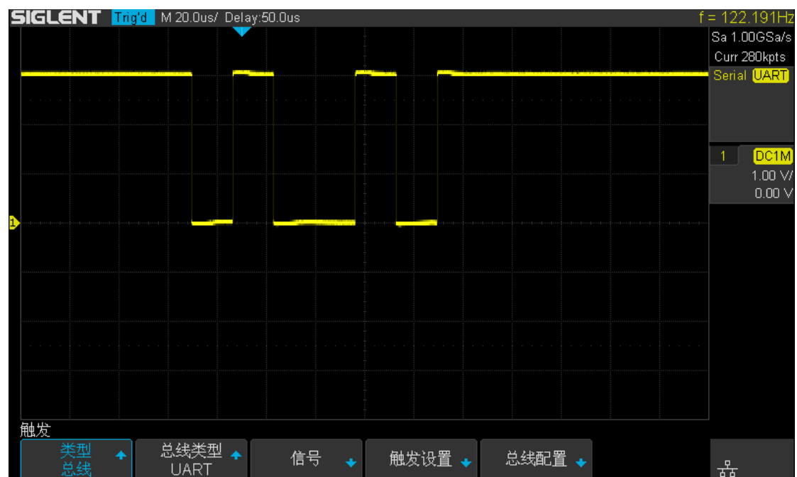
图 69 UART 触发
