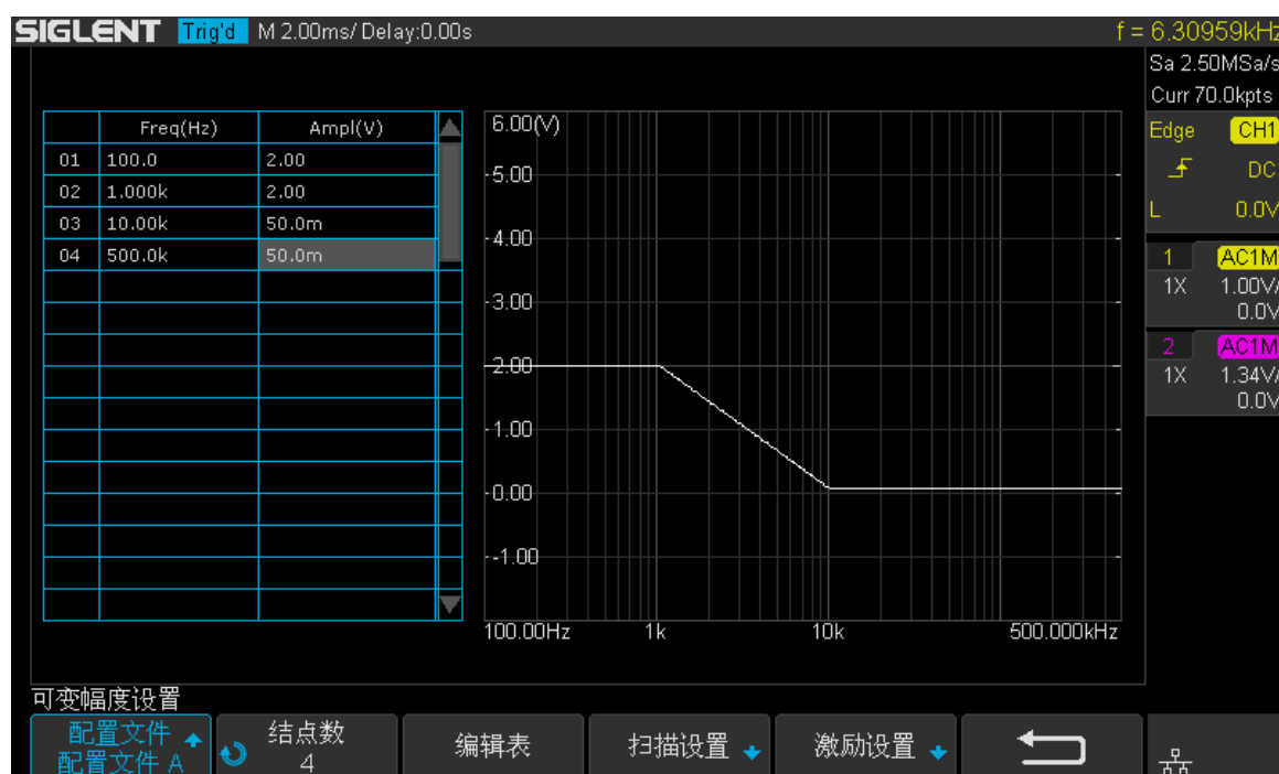
图 172 可变幅度的编辑表菜单
