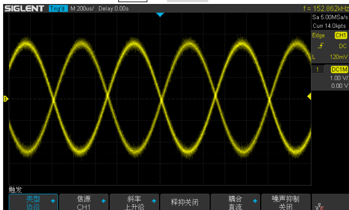
图 36 噪声抑制关闭
