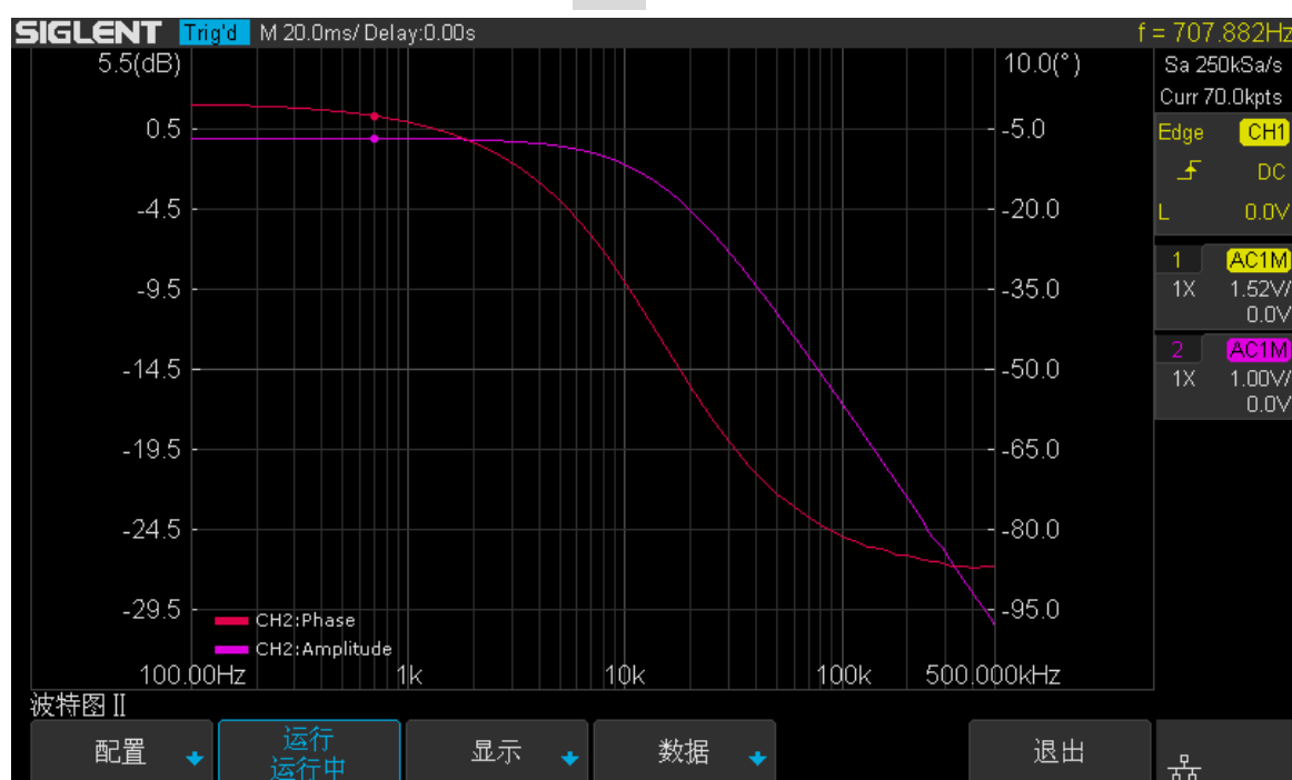
图 174 可变幅值下波特图扫描曲线
