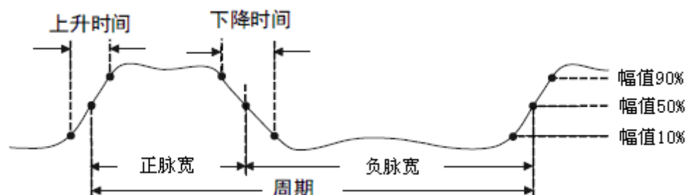
图 107 时间参数示意图
