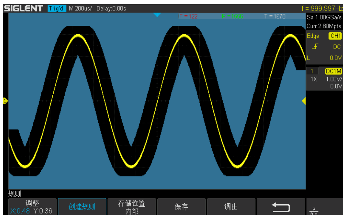
图 143 设置水平调整和垂直调整
