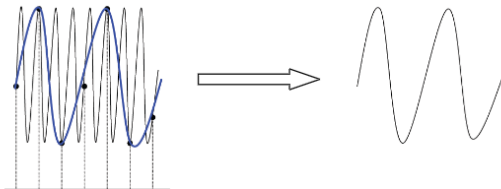
图 27 波形混叠
