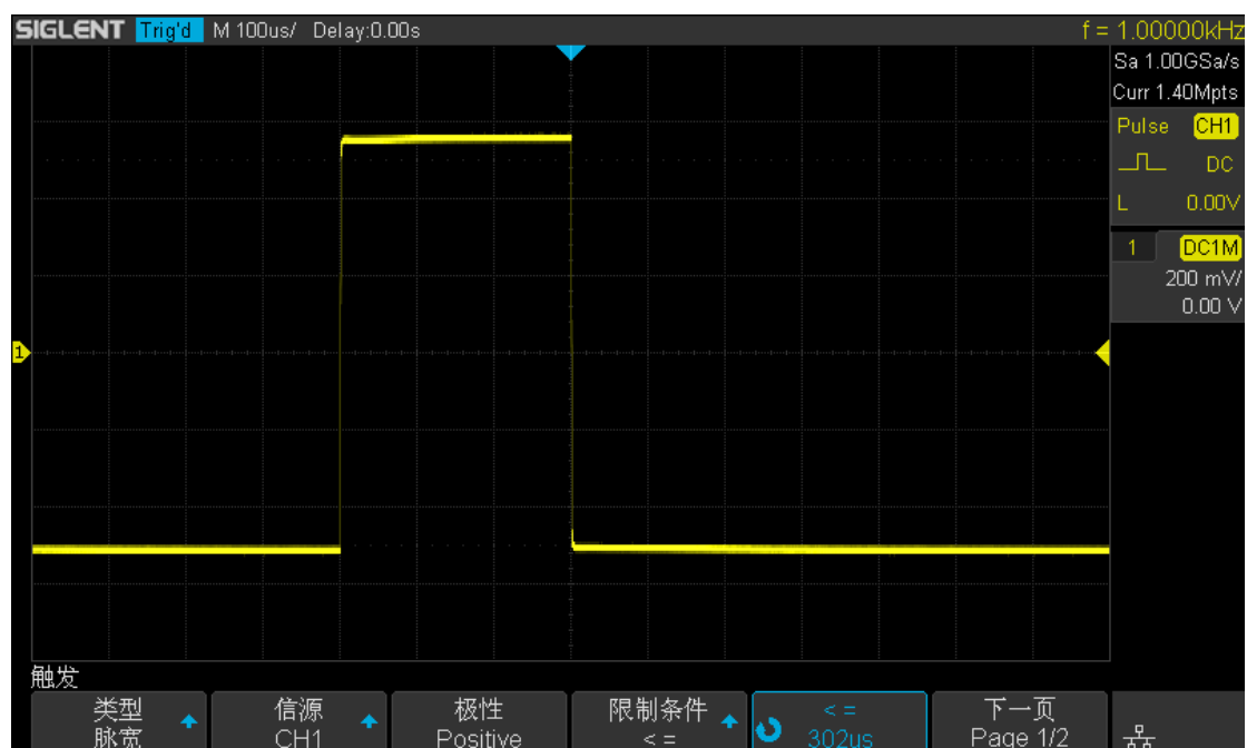
图 40 脉宽触发
