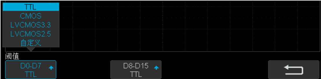
图 124 阈值设置菜单
