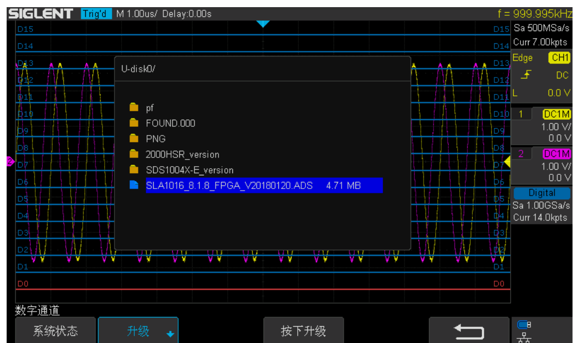
图 128 数字通道固件升级界面
