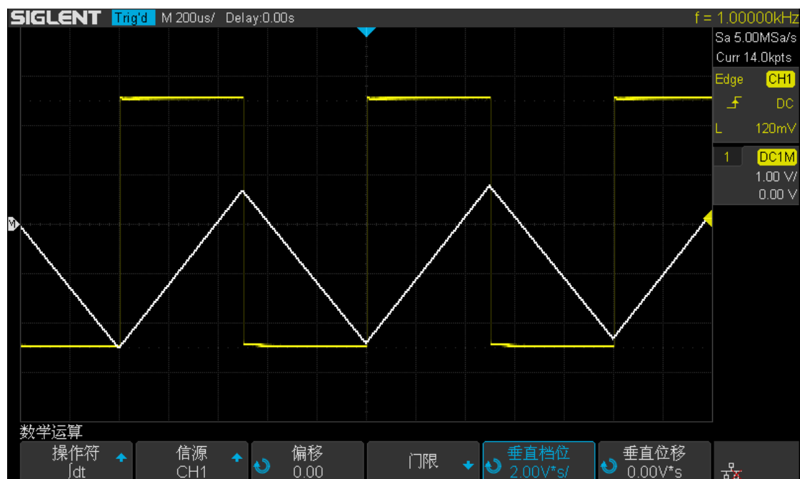
图 98 无 DC 偏移校正（积分运算）
