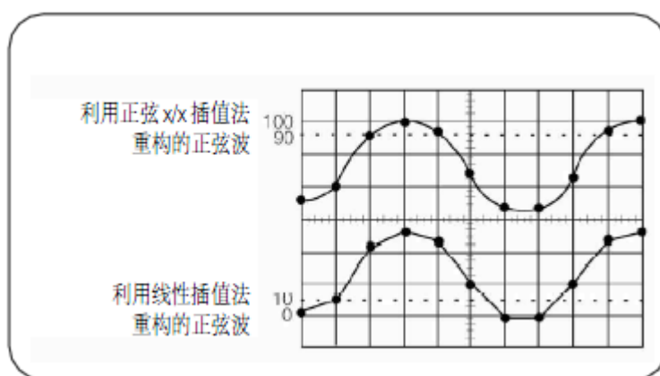
图 29 差值方式对比
