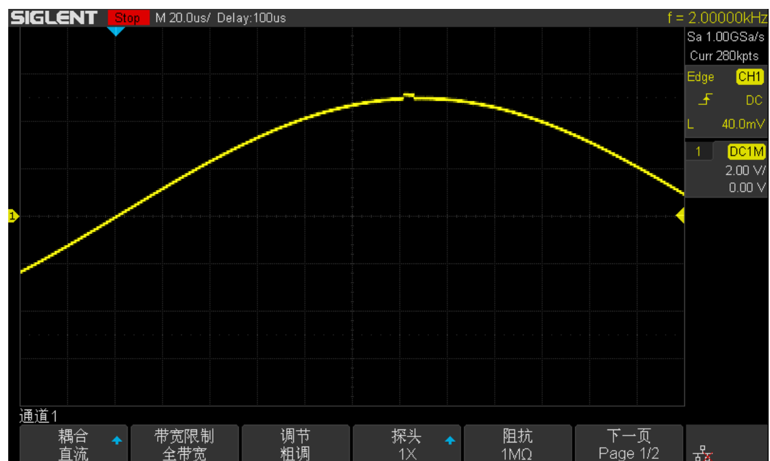
图 19 扩展后的毛刺正弦波
