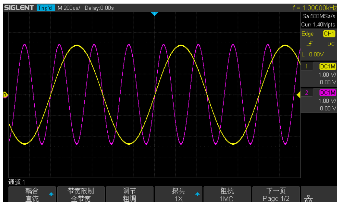
图 16 通道波形图
