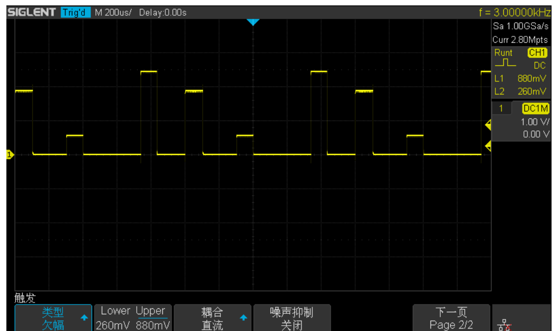
图 47 欠幅脉冲触发
