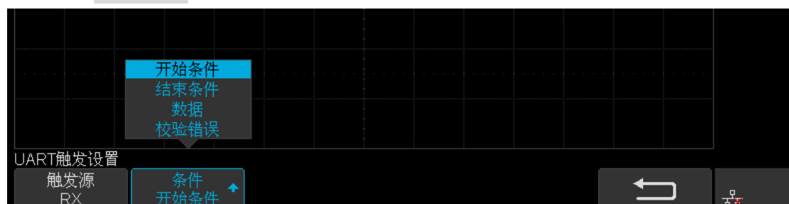
图 67 UART 触发条件
