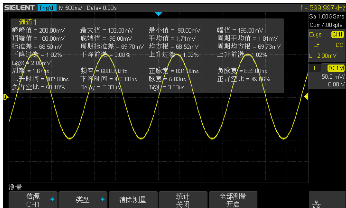
图 110 全部测量
