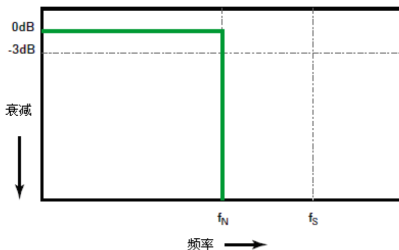
图 24 理论上的砖墙频率响应
