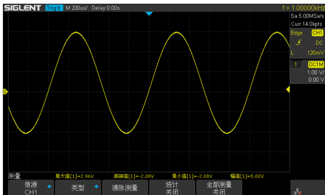
图 108 自动测量（4 个参数）
