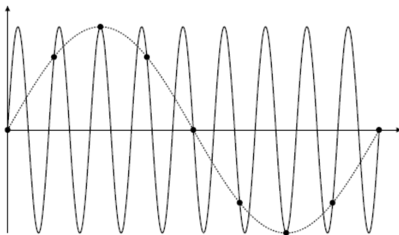
图 23 采样混叠
