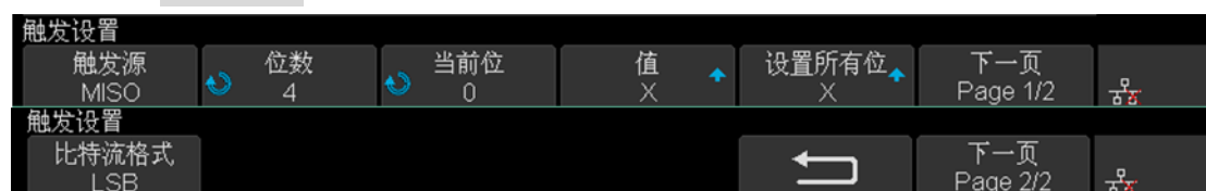
图 61 SPI 触发设置菜单
