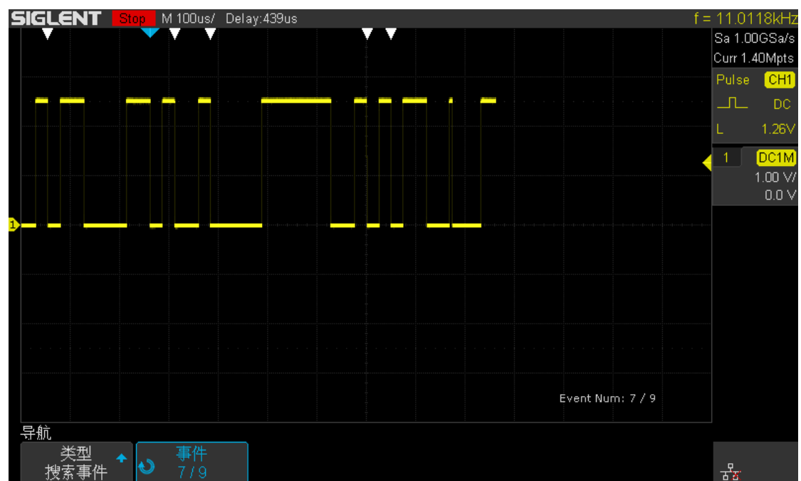
图 157 搜索事件导航
