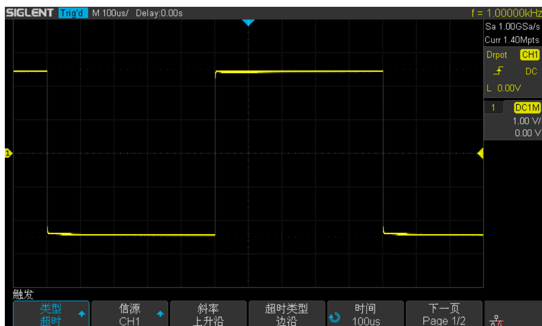
图 45“边沿”超时触发
