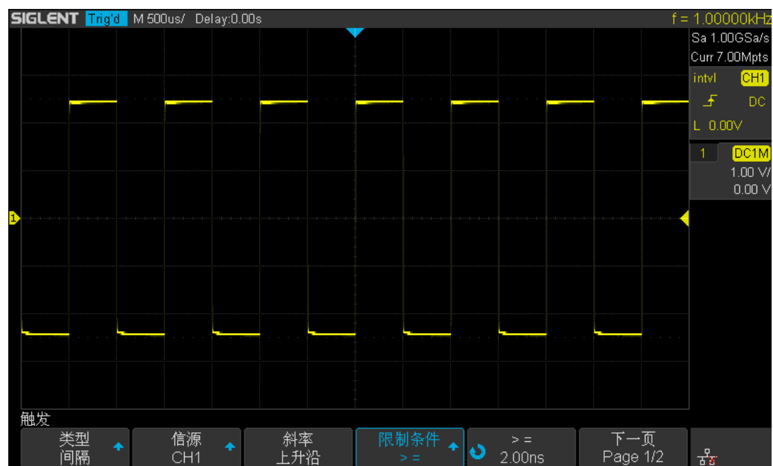
图 44 间隔触发
