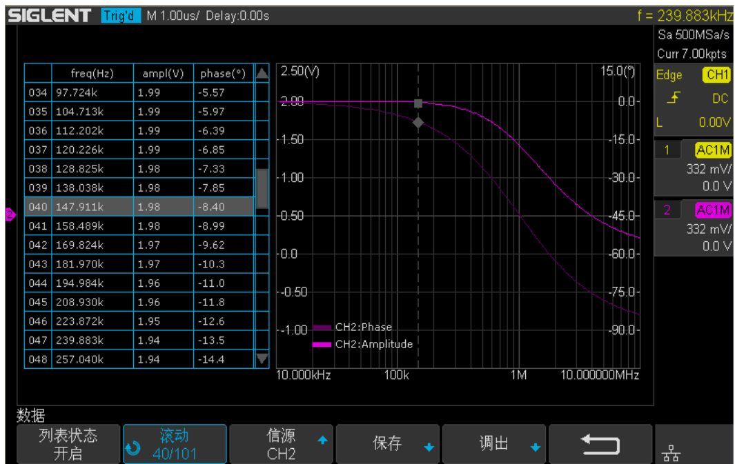
图 163 波特图列表
