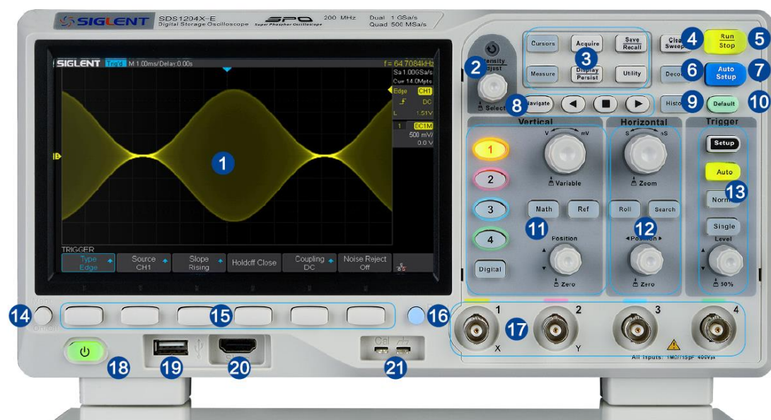
图 9-4 通道机型前面板总览
